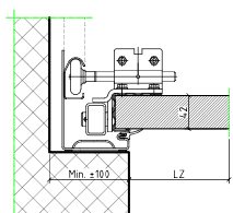
Montant affleuré
