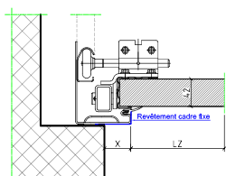
Montant décalé
