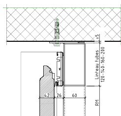
Faux linteau en tube
