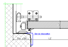
Profils de rénovation
