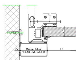
Pose entre murs
