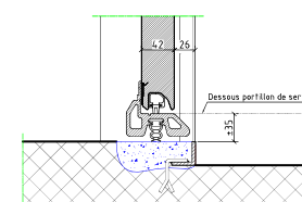
Portillon avec seuil
