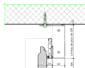
Faux linteau en tôle pliée
