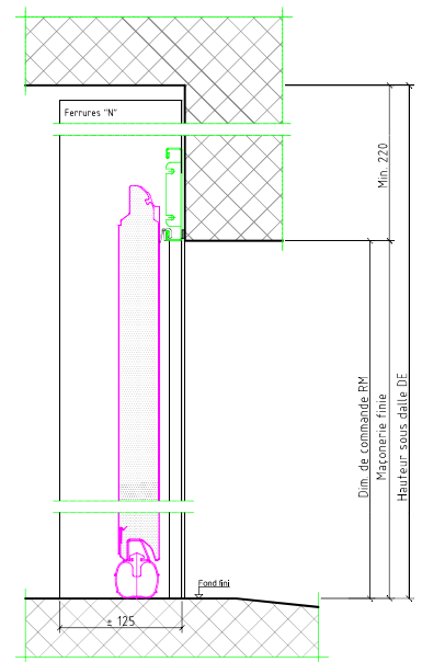
Coupe verticale
