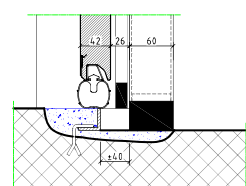
Seuil inox
