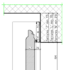
Faux linteau standard
