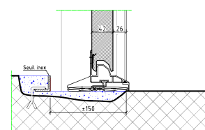
Portillon sans seuil
