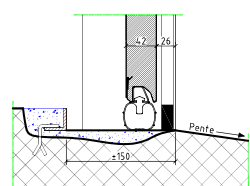
Seuil inox en retrait
