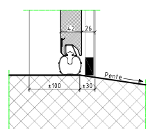
Sans seuil standard
