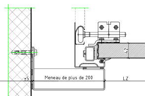
Pose entre murs
