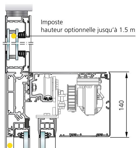
SL 35-S / SL 45-S Caisson d'entraînement 140 mm avec partie latérale et profil porteur
