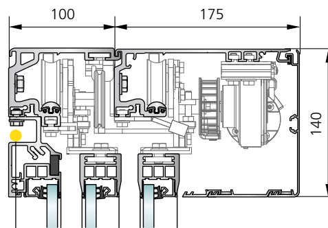
SL 35-T Caisson d'entraînement 140 mm télescopique (possible avec profil porteur)
